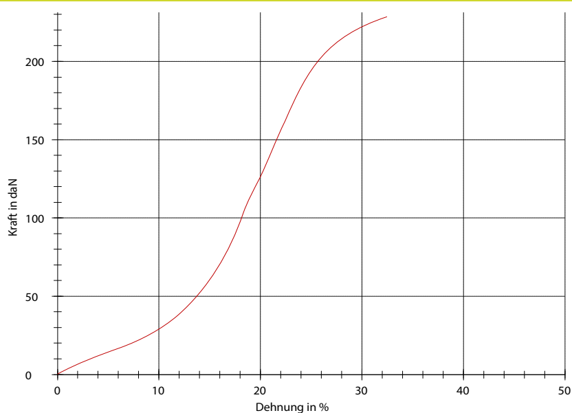
Kraft-Dehnungs Diagramm beispielhaft 2 6798 210 | Force-elongation diagram exemplified by 2 6798 210
